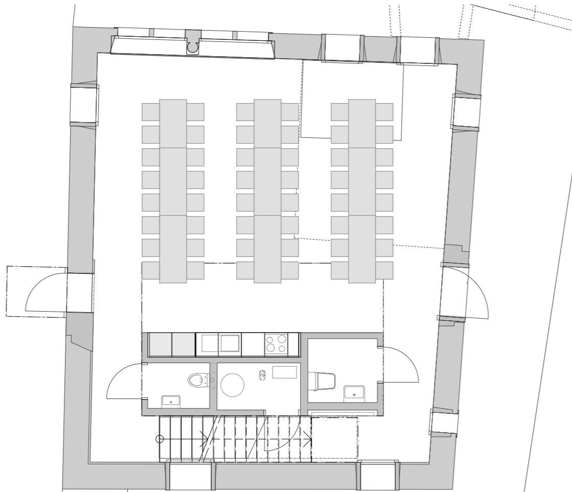
Erdgeschoss: 44 Plätze
