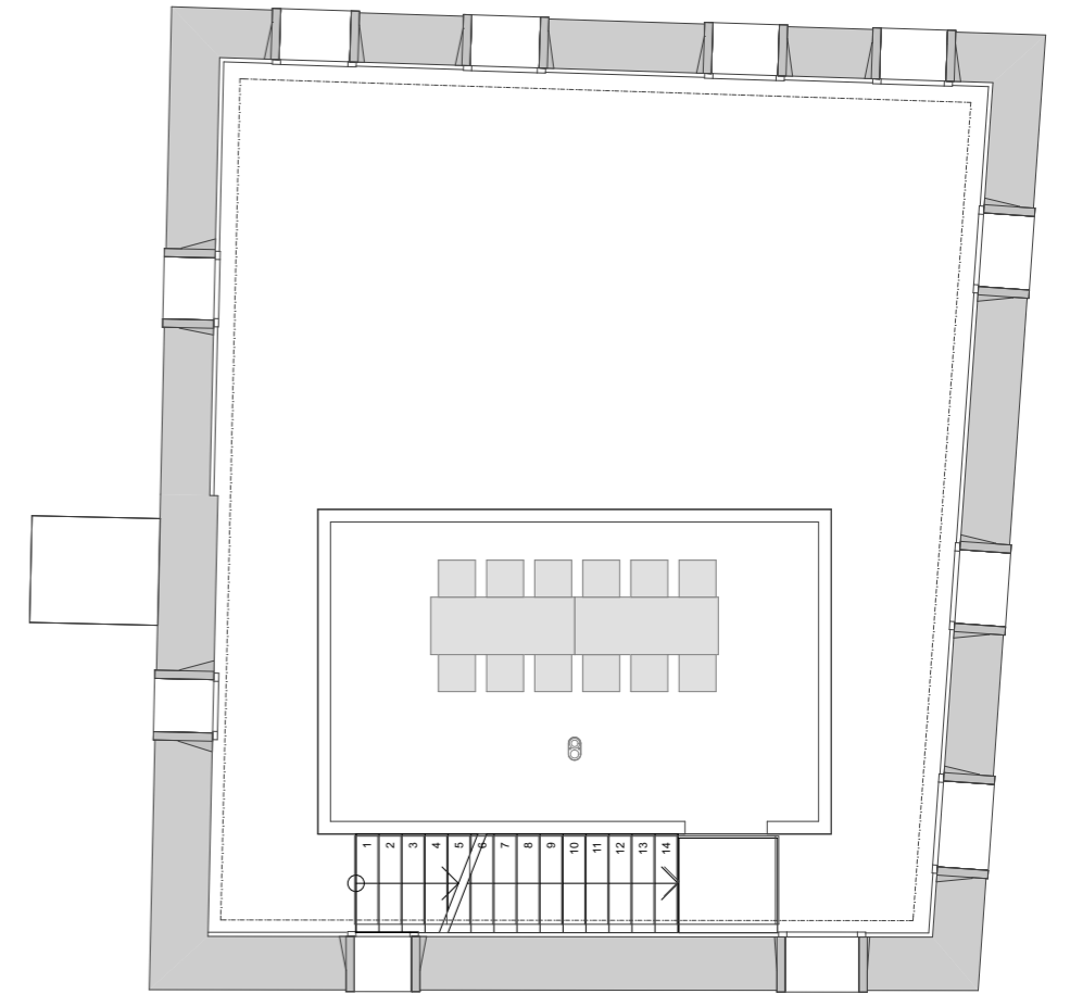
Obergeschoss: 12 Plätze
