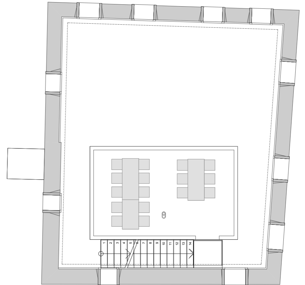
Obergeschoss: 16 Plätze
